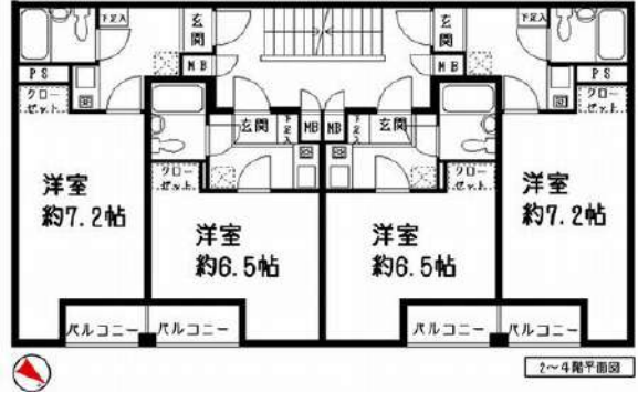
【間取り図】
