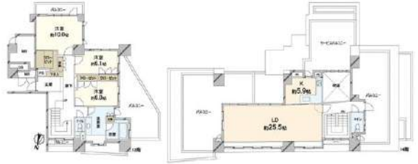
【間取り図】
