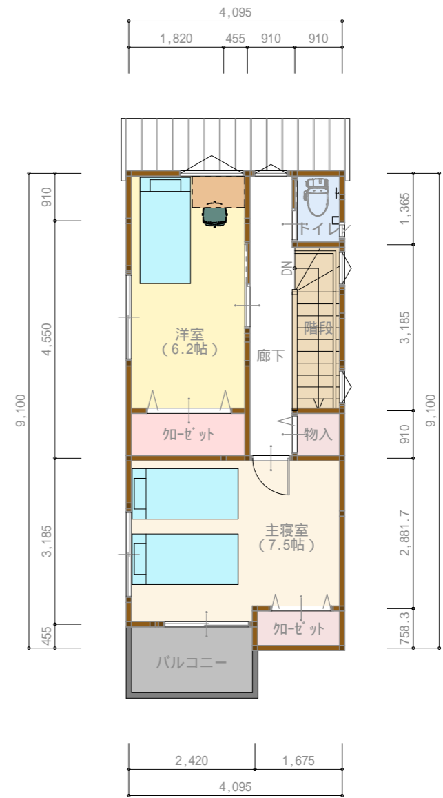
3階 平面図 S:1/100
