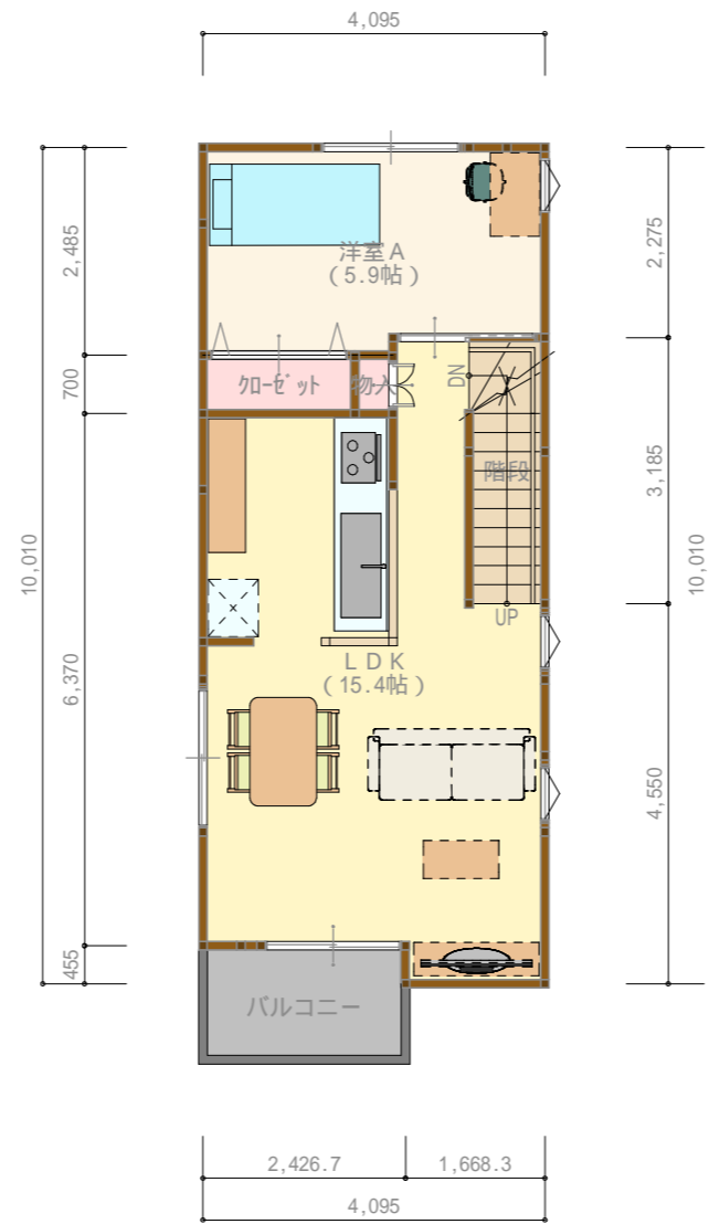
2階 平面図 S:1/100
